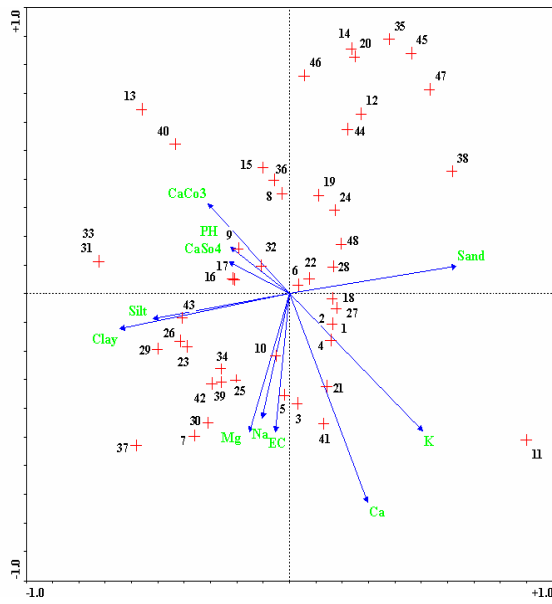
نمودار ۴- رابطه‌ی فاکتورهای خاک و سری کوادرات‌ها در روی محوره‌ای رسته‌بندی y = 3 و x = 2 به روش CCA
