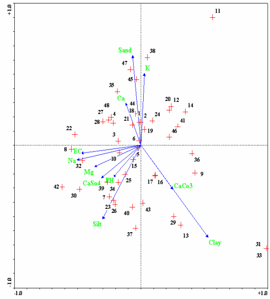
نمودار ۲- رابطه‌ی فاکتورهای خاک و سری کوادرات‌ها در روی محوره‌ای رسته‌بندی y = 2 و x = 1 به روش CCA
