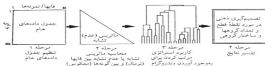
شکل ۲- مراحل طبقه‌بندی با استفاده از آنالیز خوشه‌ای (مصدقی، ۱۳۸۰)
