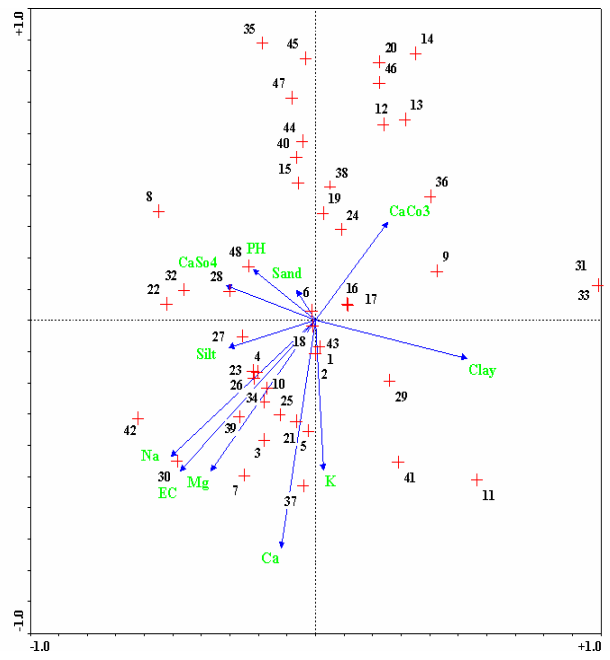
نمودار ۳- رابطه‌ی فاکتورهای خاک و سری کوادرات‌ها در روی محوره‌ای رسته‌بندی y = 3 و x = 1 به روش CCA
