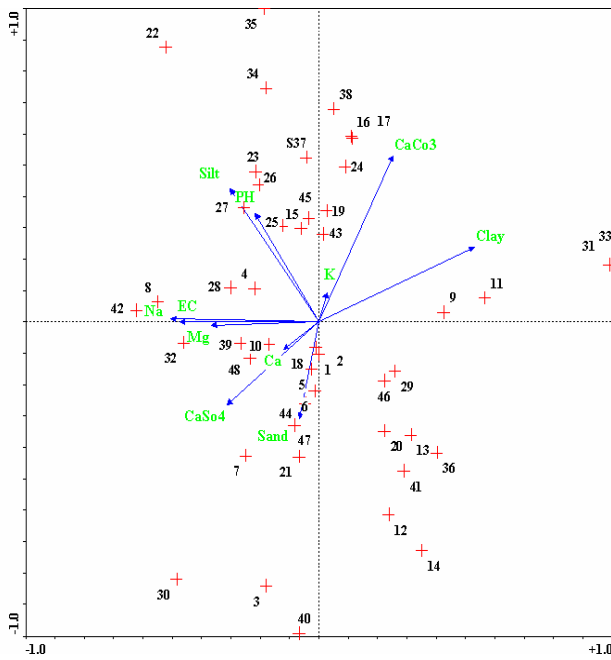
نمودار ۵- رابطه‌ی فاکتورهای خاک و سری کوادرات‌ها در روی محوره‌ای رسته‌بندی y = 4 و x = 1 به روش CCA
