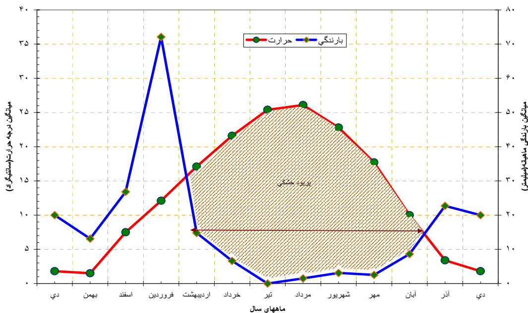
شکل ۱- منحنی آمپروترمیک منطقه طرح
