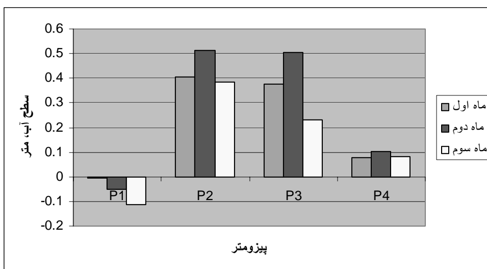
شکل ۱۱- نمودار سطح آب زیرزمینی دشت گرهایگان در سه ماه بعد از سیلاب منطبق با داده های بده.
