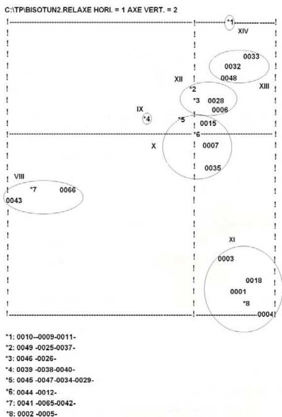
شکل ۴- محورهای ۱ و ۲ AFC قطعات نمونه (تجزیه و تحلیل مرحله
