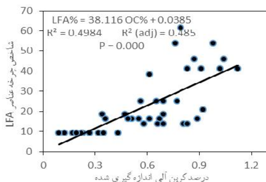
شکل ۴- رابطه رگرسیونی شاخص چرخه عناصر بین اندازه‌گیری آزمایشگاهی و روش LFA
