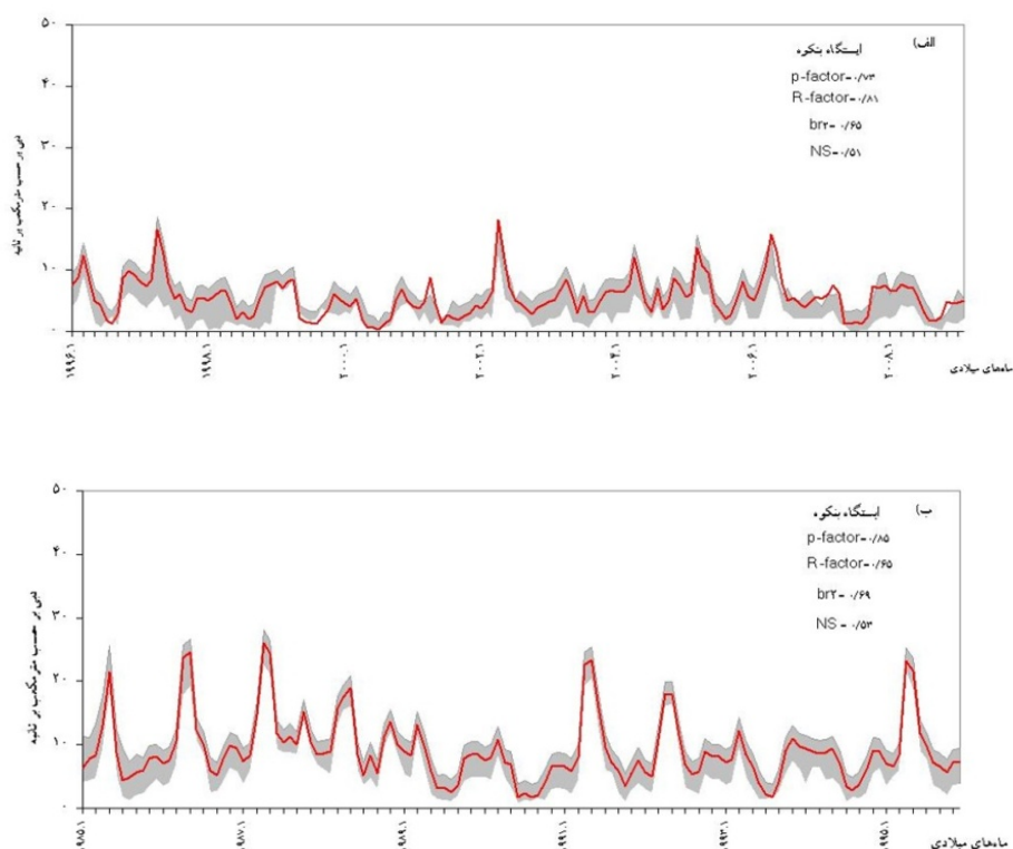
شکل ۲- مقایسه داده‌های واقعی دبی (خط قرمز) با داده‌های شبیه‌سازی شده (باند اطمینان در سطح ۹۵٪)؛ واسنجی داده‌های دبی در مدت زمان ۱۴ ساله (الف)، اعتبارسنجی داده‌ها در مدت زمان ۱۰ ساله (ب)
