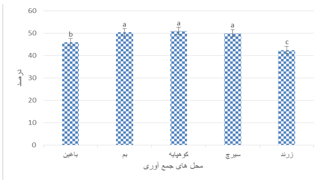
شکل ۱- مقایسه میانگین درصد استقرار در جمعیت‌های ( Fortuynia bungei ) جمع‌آوری شده از مناطق مختلف استان کرمان
