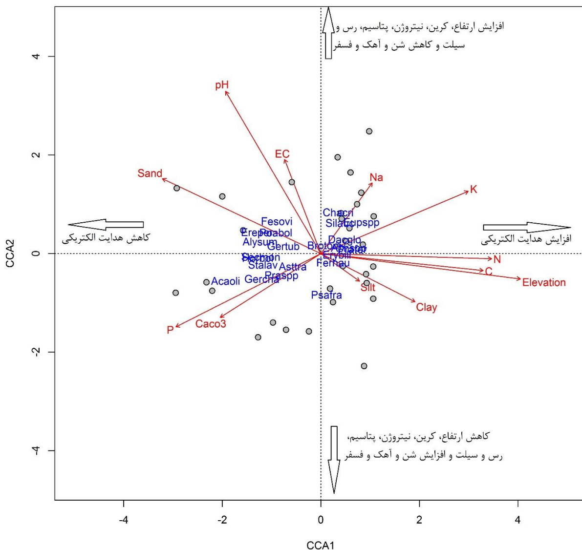
شکل ۲- دیاگرام دوپلاتی گونه-محیط حاصل از رج بندی CCA
