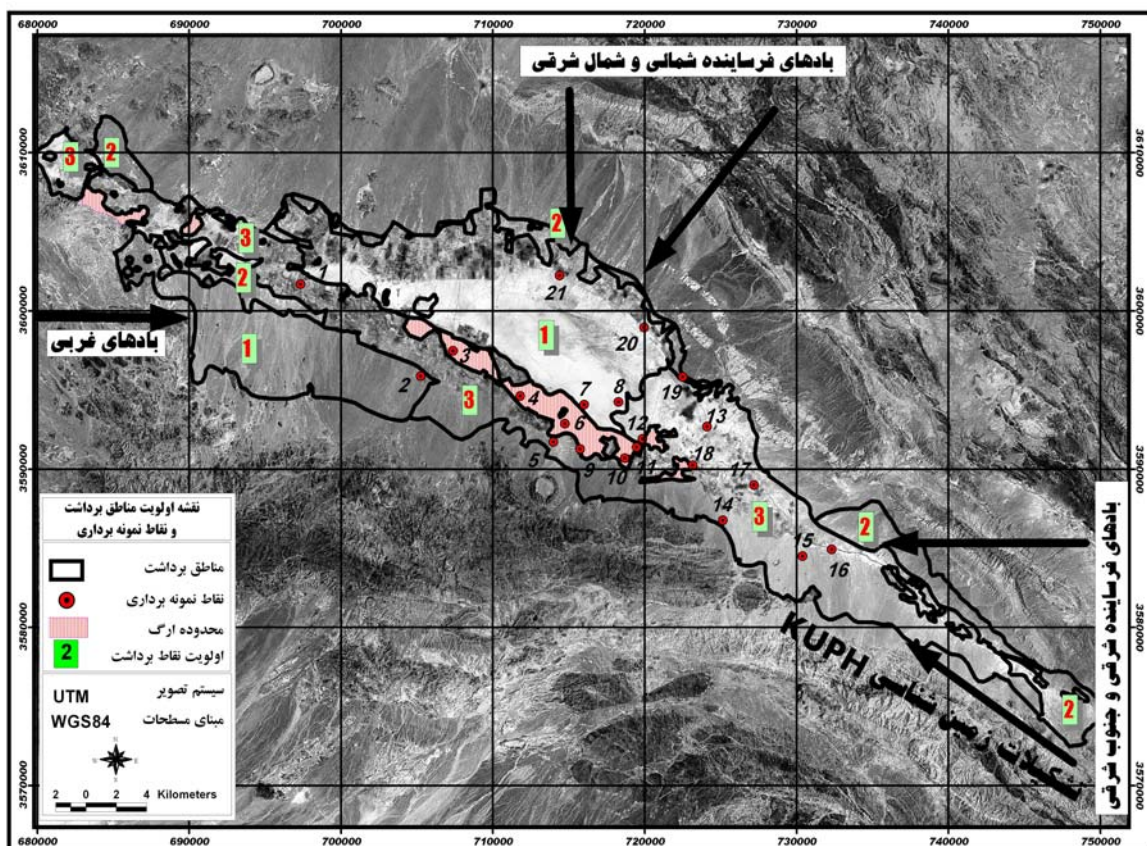
شکل ۸ - نقشه اولویت بندی مناطق برداشت رسوبات بادی
