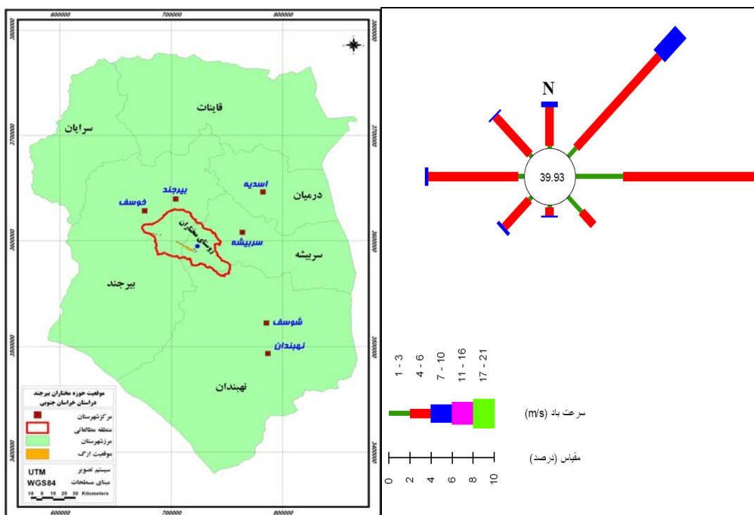
شکل ۲- گلباد سالیانه ایستگاه سینوپتیک بیرجند
