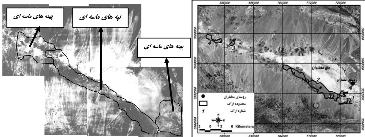
شکل ۴ - مقایسه محدوده‌های از ارگ دشت مختاران در دو دوره زمانی ۱۳۳۴ و ۱۳۸۴
