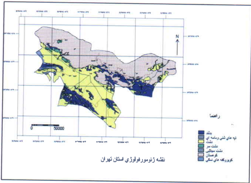
نقشه شماره ۱- رخساره های ژئومورفولوژیکی خاص بیابان استان تهران
