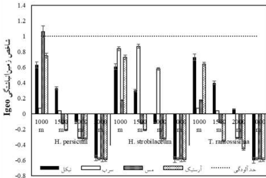
شکل ۲- شاخص زمین انباشت چهار عنصر سنگین در سه گونه هالوفیت مورد بررسی در چهار فاصله از معدن. حد آستانه آلودگی استاندارد به وسیله خط نقطه چین مشخص شده است. ستون‌های با همپوشانی یکسان بر اساس برآورد خطای استاندارد (±SE) تفاوت معنی دار ندارند.
